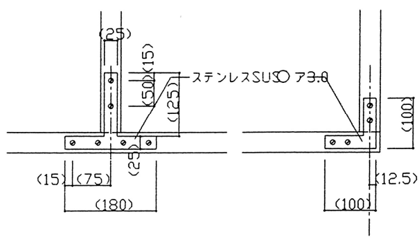
上部補強金物
