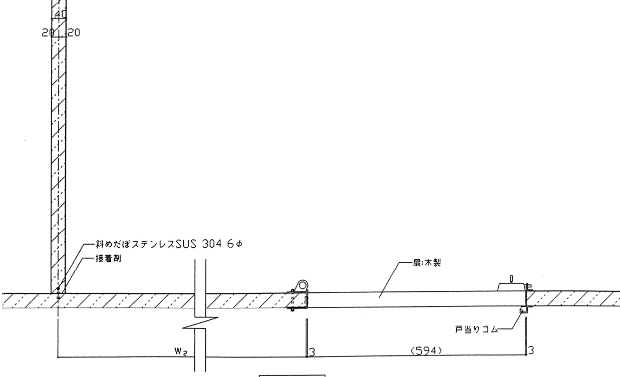
平面図
